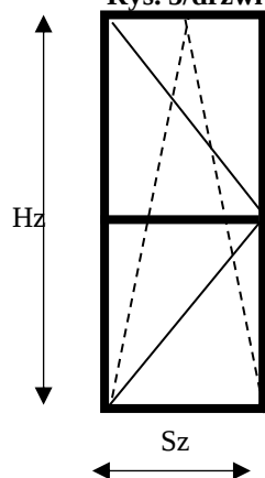
Rys. 5/drzwi balkonowe/
